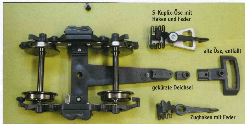
Explosionsdarstellung der Umrüstung eines Kiss-Drehgestells.
