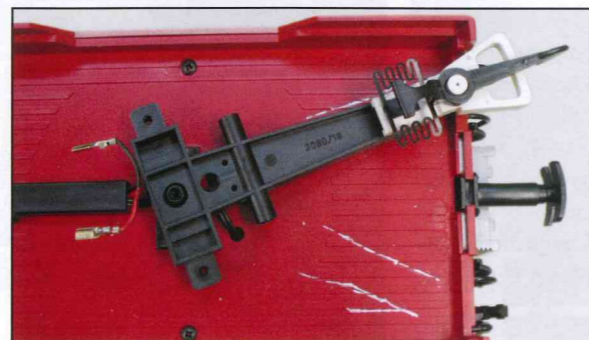
Die S-Kuplix-Öse ermöglicht den vollen Schwenkbereich auch bei Verwendung der kurzen US-Wagendeichsel oder einer gekürzten RhB-Deichsel. Der Puffer ist noch ungekürzt.
