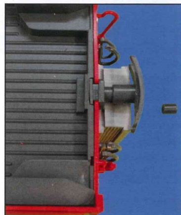
Unverzichtbar bei Kiss (Bild oben) und LGB: Die Mittelpuffer müssen gekürzt werden.
