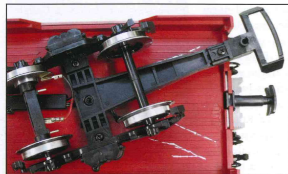
Blick unter einen LGB-Panoramawagen im Lieferzustand. Der Schwenkradius der Deichsel ist weiß markiert.
