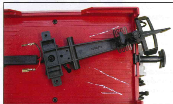
Einsatz der kurzen LGB-Deichsel 3080 / 19 eines US-Plattformwagens von LGB. Der Schwenkbereich verkleinert sich, weil die breite Standardöse am Wagenkasten aneckt.
